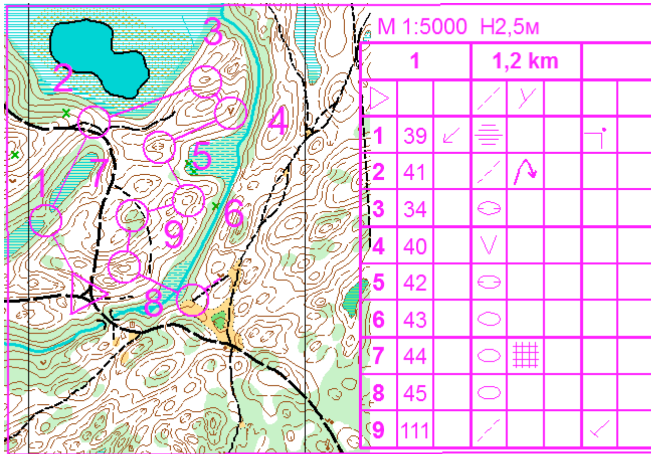
Образец дистанции для групп М/Ж 9,10,12 дисциплина рельеф 13 июля.
